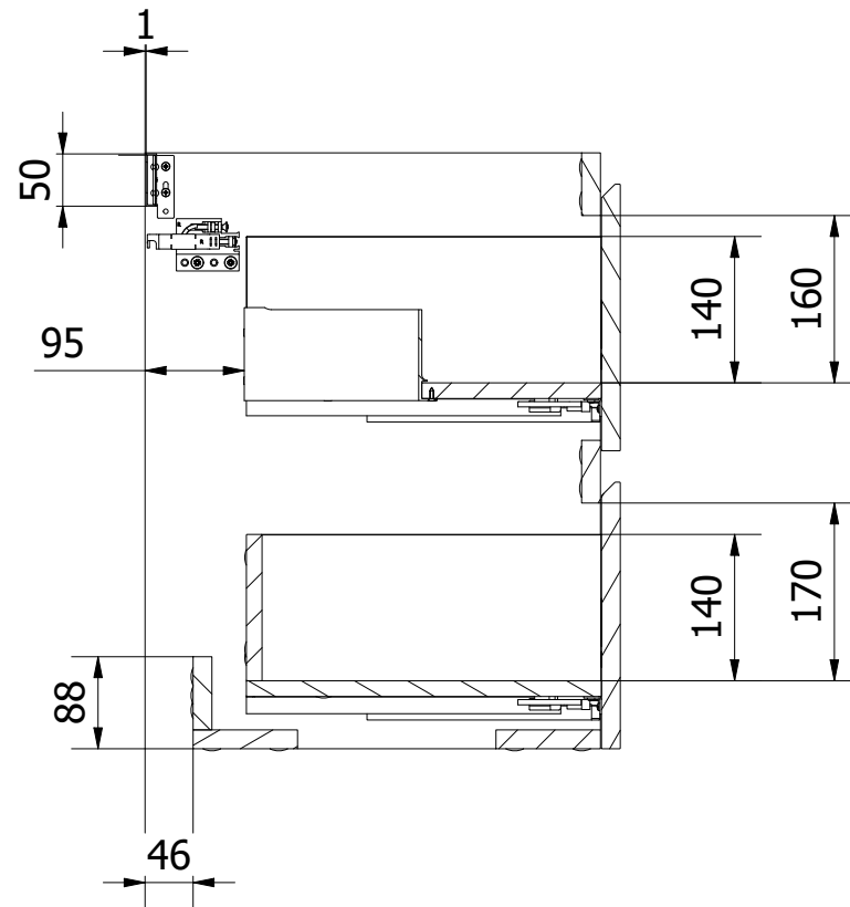
A-A ( 1 : 8 )
